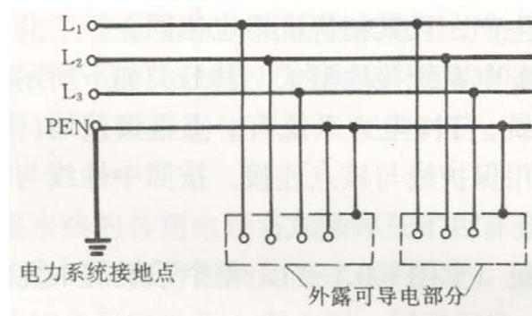
图 7.0.1-1 TN-C 系统
