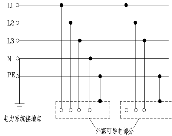
图 7.0.1-3 TN-S 系统
