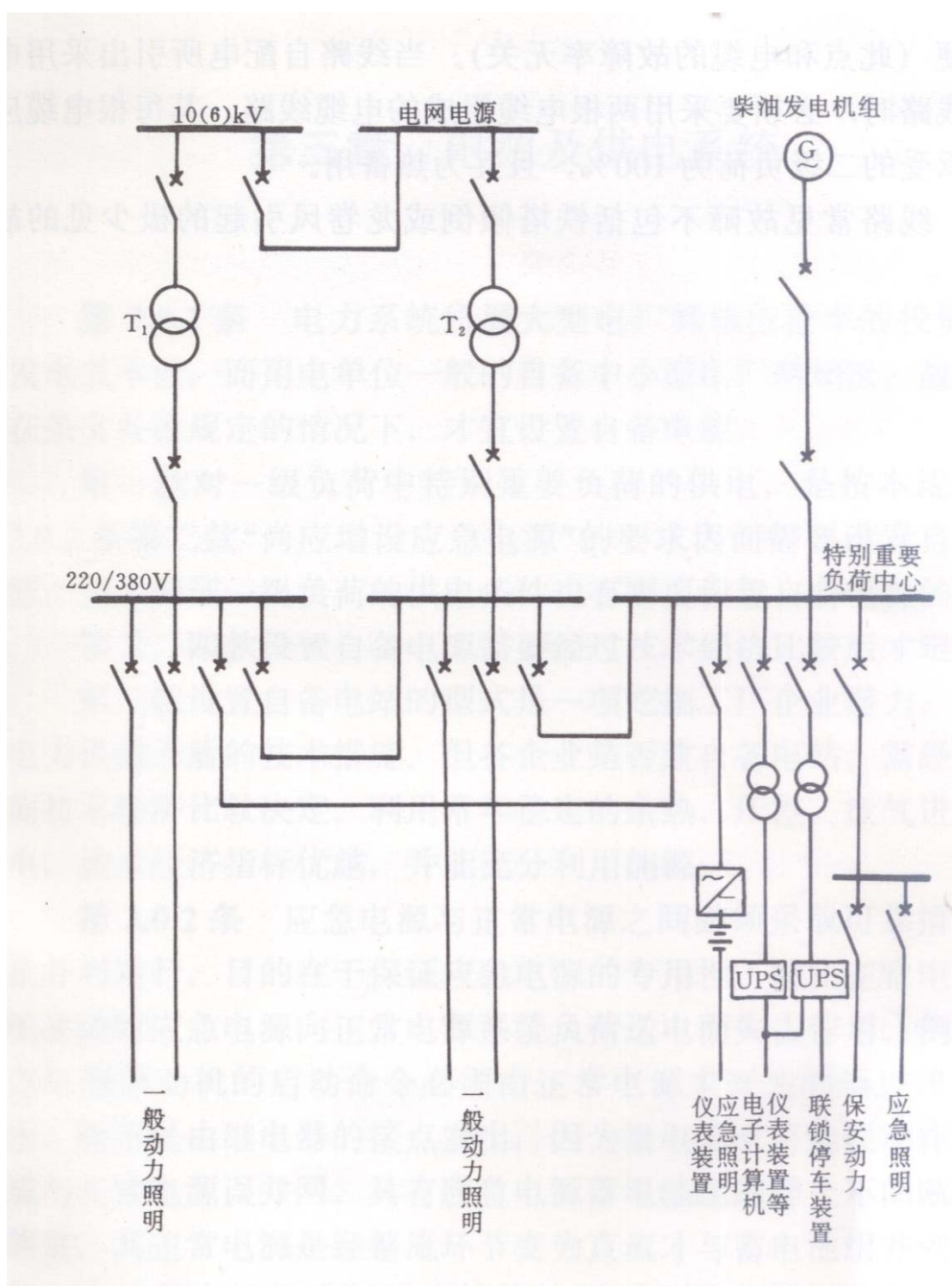
图 3.0.5 应急电源接线示例
