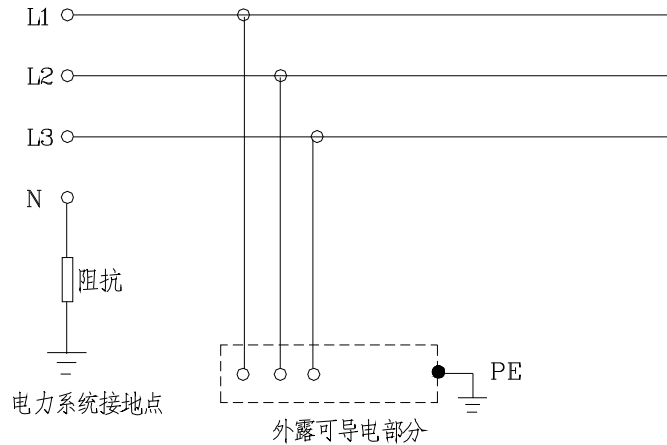
图 7.0.1-5 IT 系统
